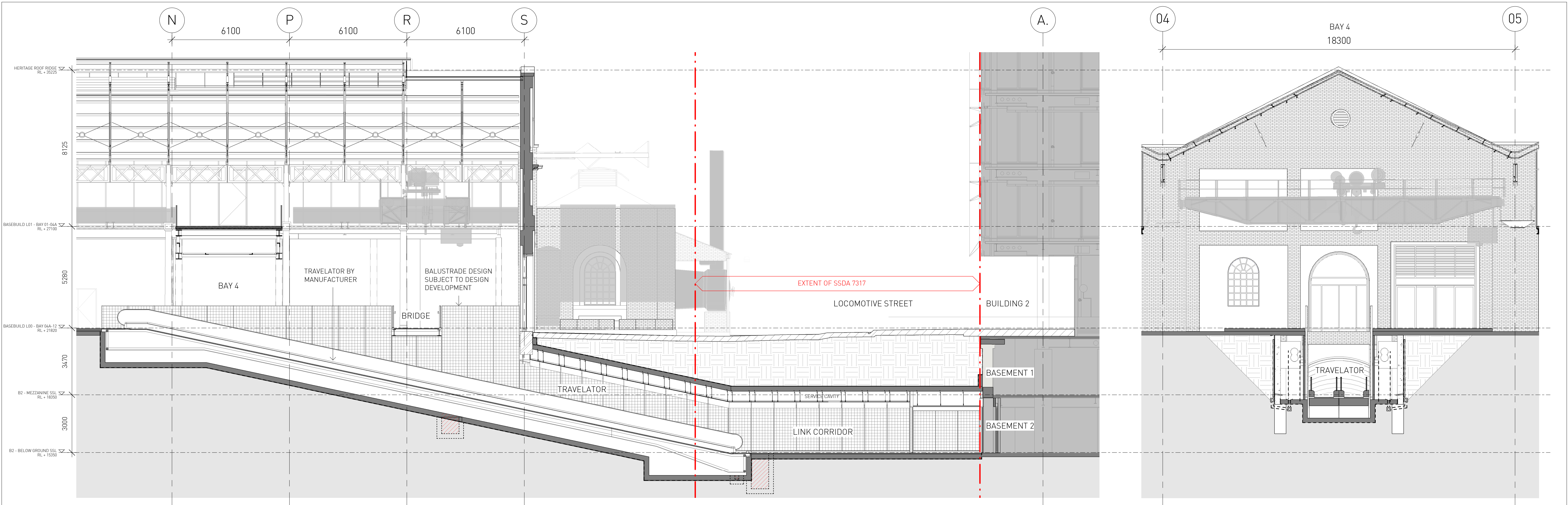
1 Long Section 1 : 100 2 Short Section 01 1 : 100 3 Short Section 02 1 : 100 4 Perspective Section
